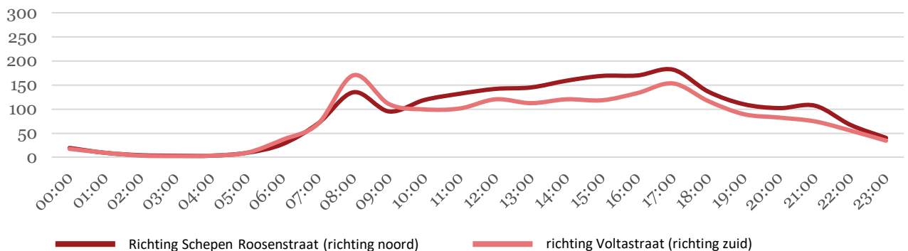
Verloop over de dag: aantal motorvoertuigen per uur (werkdag)
