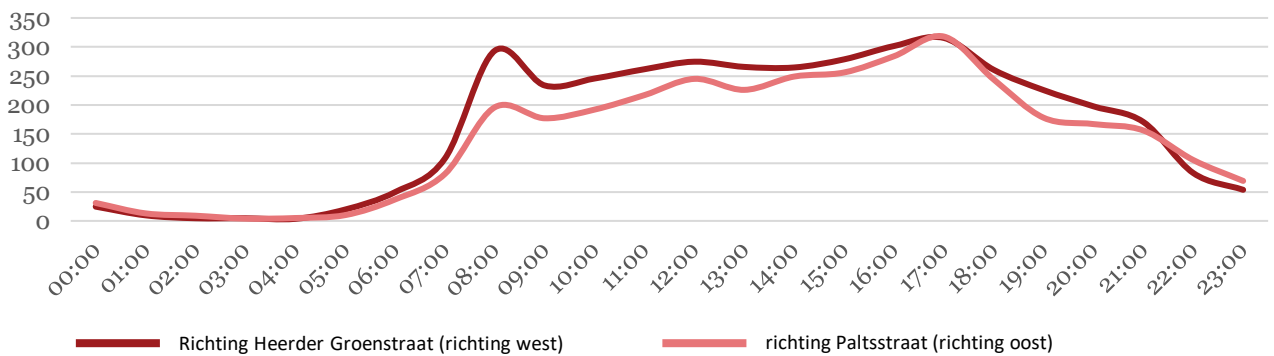
Verloop over de dag: aantal motorvoertuigen per uur (werkdag)
